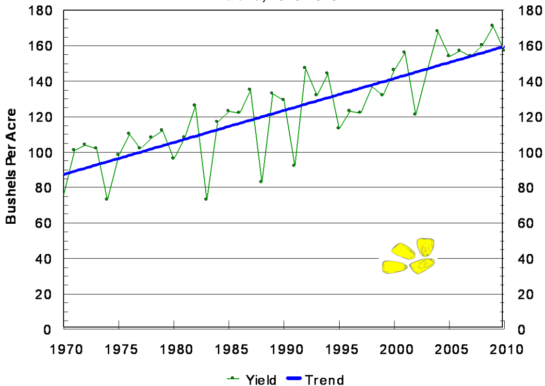
Corn Yield Trend Indiana, 1970-2010
